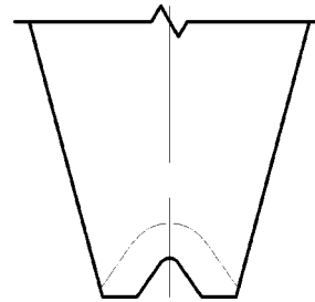
OSG7 DEEP V GROOVE STYLE
