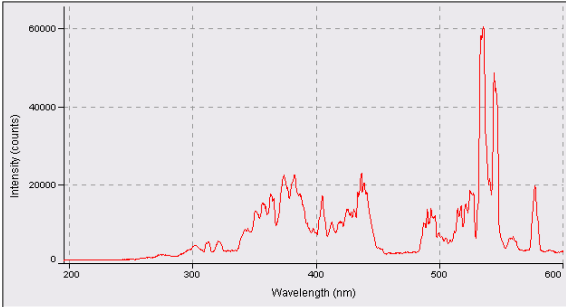
UV SOURCE RANGE: 200 – 600nm
